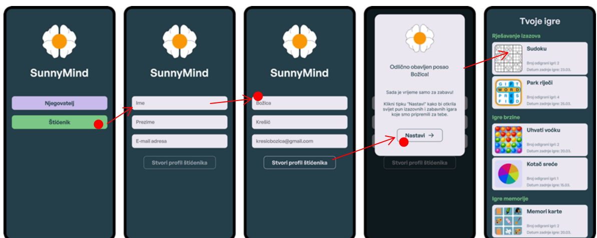
Slika 49. Prikaz ulogiravanja u aplikaciju sa strane štitenika
