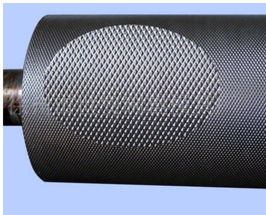
Slika 3. Aniloks cilindar
