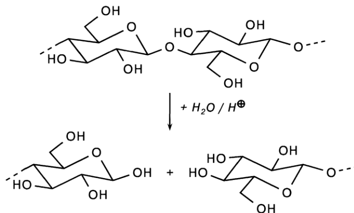
Slika 2. Hidrolitička degradacija glikozidnih veza u celulozi [7]
