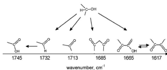
Slika 5. Produkti oksidacije celuloze i njihove vibracije u IR spektru [16]
