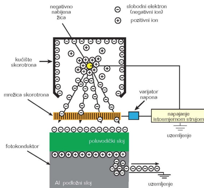
Slika 5. Princip negativnog nabijanja (Izvor: I. Majnarić, Studija indirektno elektrografije, doktorska disertacija, 2007.)
