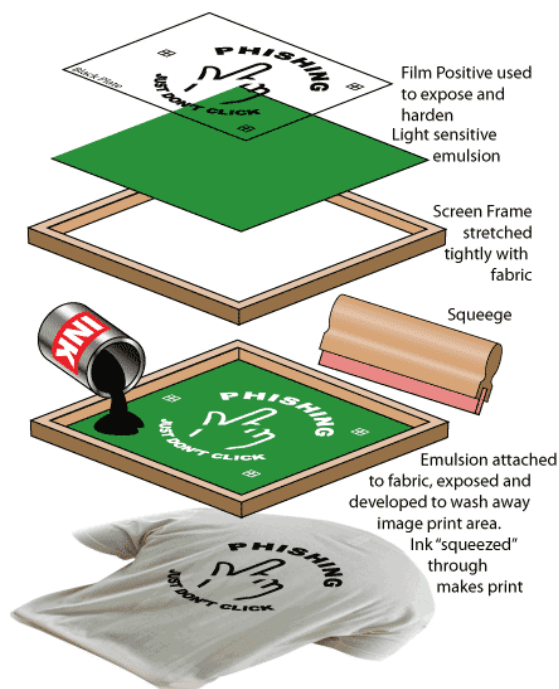
Slika 2. Proces sitotiska
