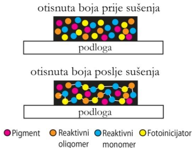
Slika 19. Fotopolimerizacija
