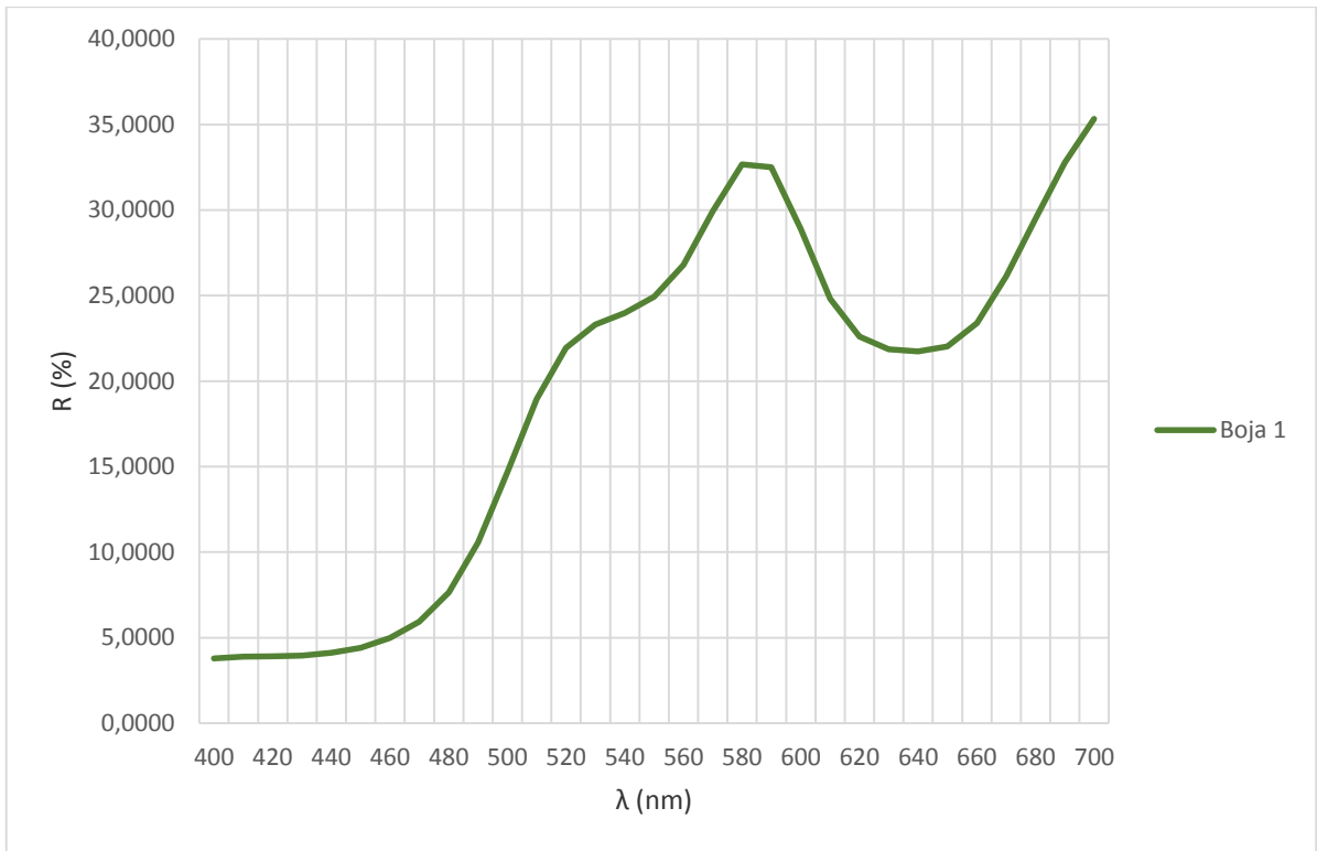
Slika 28 Spektrofotometrijska krivulja uzorka 1
