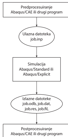
Slika 16. - Dijagram toka rada Abaqus CAE softvera [16]
