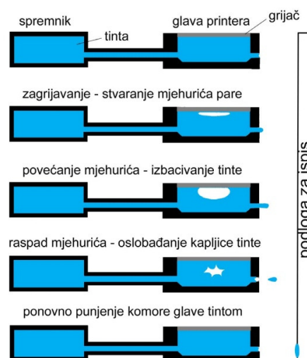
Slika 2. Termalni-bubble jet
