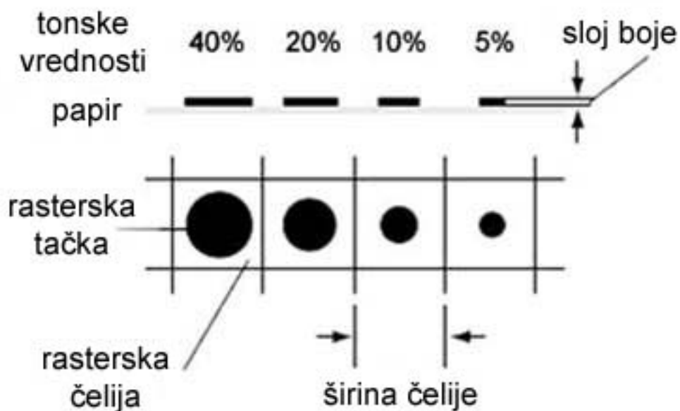
Slika 2 - Reprodukija kontinuiranog tona AM rasterom [7].
