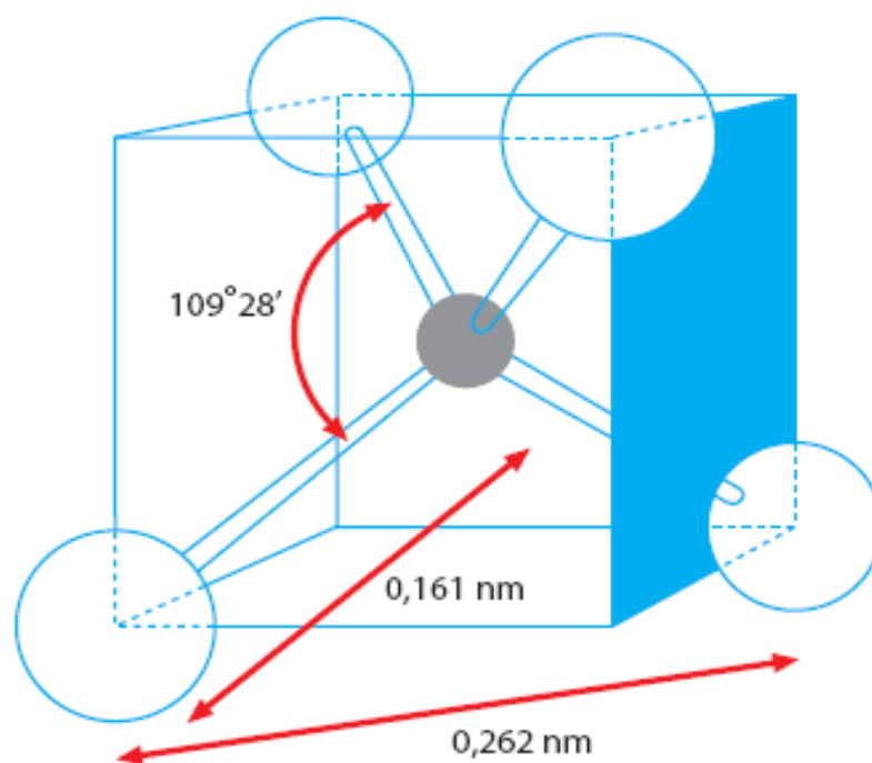
Slika 1. Primarne strukturne jedinice [ (\text{SiO}_4)^{4-} i (\text{AlO}_4)^{5-} tetraedri] zeolita. U izoliranoj strukturnoj jedinici \text{SiO}_4 , ukupni naboj je 4. Zamjena atoma silicija aluminijem dovodi do ukupnog naboja 5-. Udaljenost O-O = 0,262 nm; udaljenost Si-O = 0,161 nm; kut O-Si-O = 109^\circ 28' .
