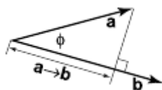
Slika 5. Projekcija vektora na drugi vektor, preuzeto iz [5]
