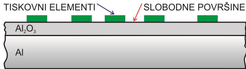
Slika 3. Monometalna tiskovna forma
