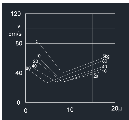
Slika 1. Utjecaj debljine sloja boje na brzinu kod koje dolazi do čupanja [3]
